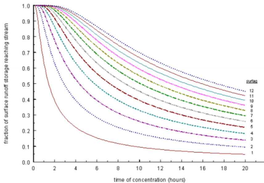
รูปที่ 3.1.4-1 ความสัมพันธ์ระหว่าง Surlag และ t conc
