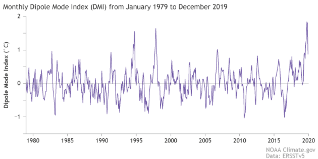
รูปที่ 2.4-1 สถานะของ Indian Ocean Dipole
