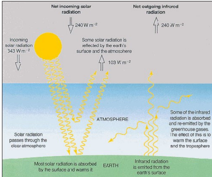
รูปที่ 1.2.1-1 ลักษณะการดูดซับและการปล่อยรังสีของโลก
