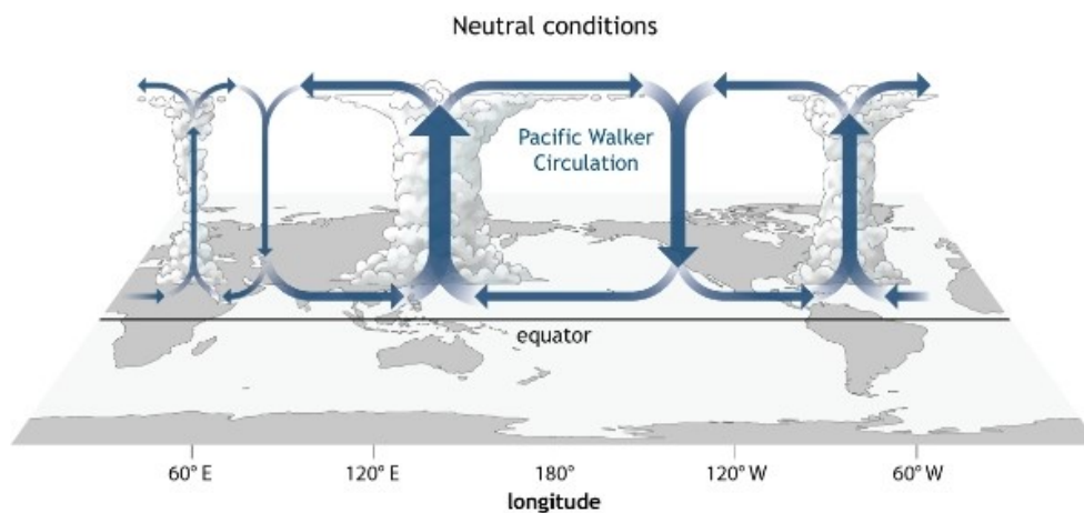
รูปที่ 2.1.1-1 ลักษณะการเคลื่อนที่ของมวลอากาศของโลก
