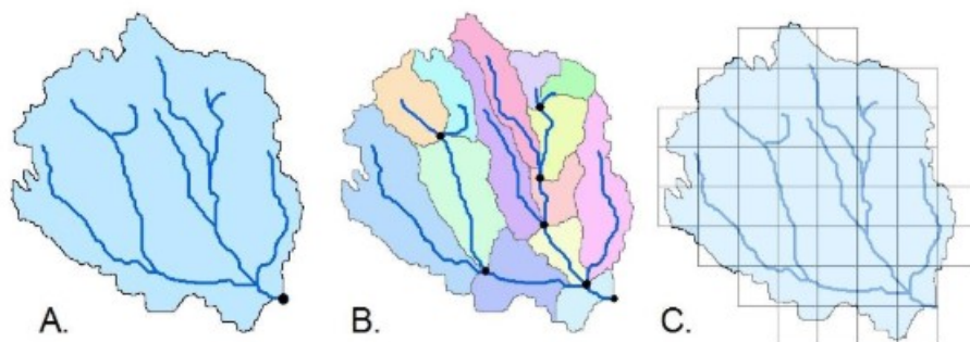
รูปที่ 6.4.1-1 การแบ่งประเภทของแบบจำลองอุทกวิทยา (Model Classification)
