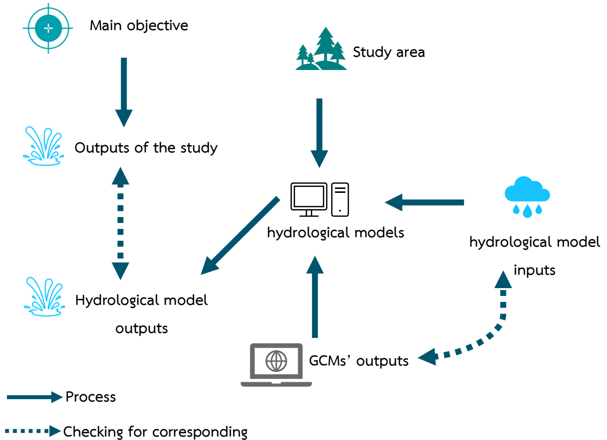
รูปที่ 6.3.4-1 การตรวจสอบแบบจำลองทางอุทกวิทยากับผลลัพธ์ของแบบ GCMs
