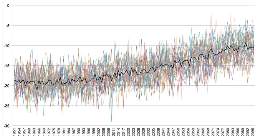
รูปที่ 3.5-1 อุณหภูมิต่ำสุดในพื้นที่หนึ่งในช่วงระหว่างปี 1951 – 2096 จากการประยุกต์ใช้แบบจำลองภูมิอากาศโลก 24 แบบจำลอง
