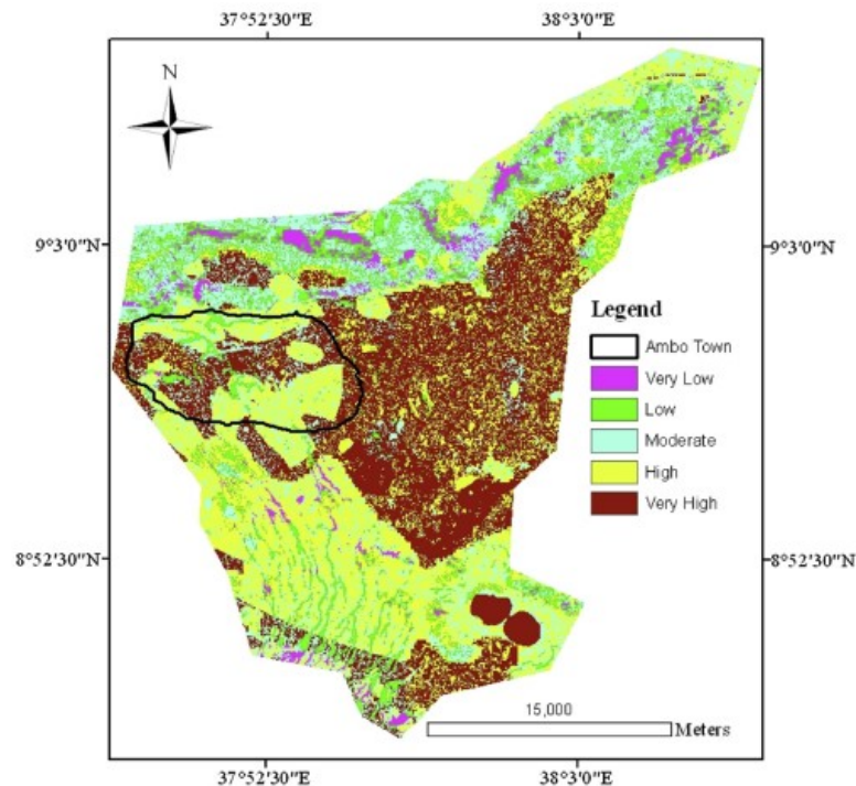
รูปที่ 7.3.2-2 ตัวอย่างแผนที่ภัยอันตรายจากน้ำท่วมจากงานวิจัยในประเทศเอธิโอเปีย
