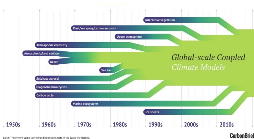
รูปที่ 3.2-1 การพัฒนาของแบบจำลอง GCM ในแต่ละช่วงเวลา
