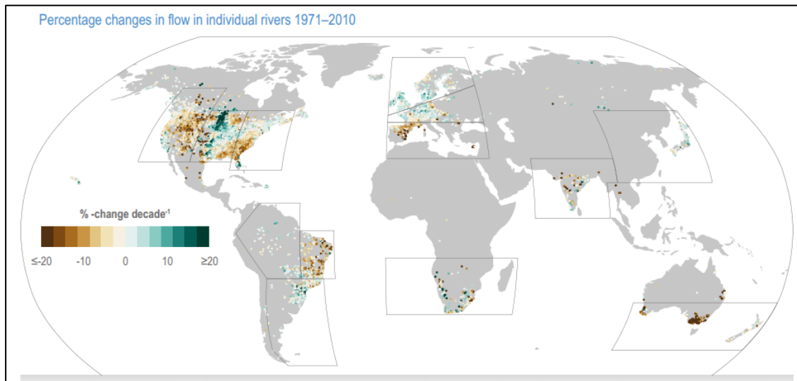
รูปที่ 6.2.1-3 การเปลี่ยนแปลงปริมาณน้ำในลำน้ำในแต่ละแม่น้ำสายหลักในช่วงระหว่างปี 1971-2010
