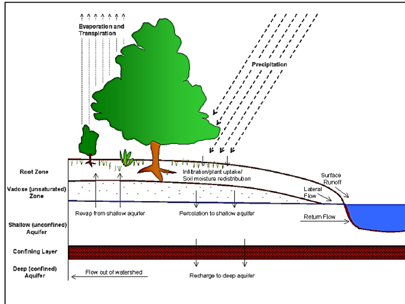
รูปที่ 2-1 วัฏจักรอุทกวิทยา
