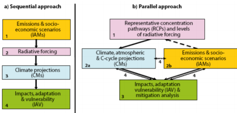
รูปที่ 4.3.1-1 ขั้นตอนการพัฒนาสถานการณ์การปล่อยก๊าซเรือนกระจก SRES (ซ้าย) และ RCPs (ขวา)
