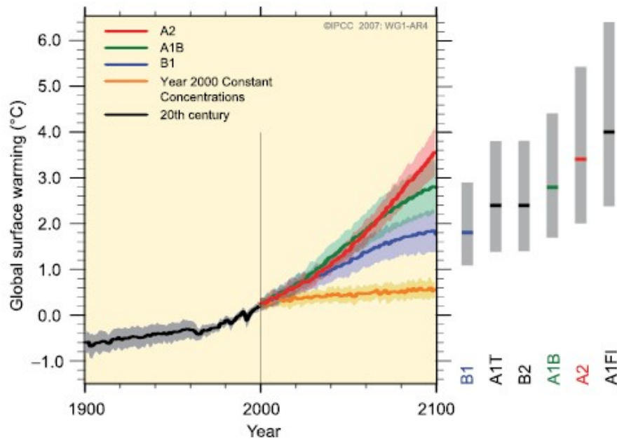
รูปที่ 4.2.2-1 แนวโน้มการเปลี่ยนแปลงอุณหภูมิสถานการณ์ A1B, A2 และ B1 ในแต่ละปี
