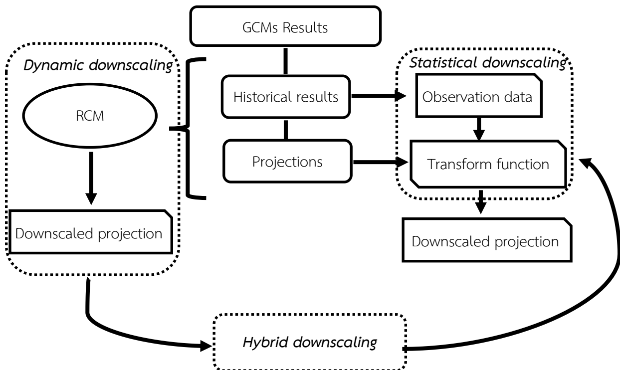
รูปที่ 5.2.3-1 กระบวนการลดมาตราส่วน 3 วิธี
