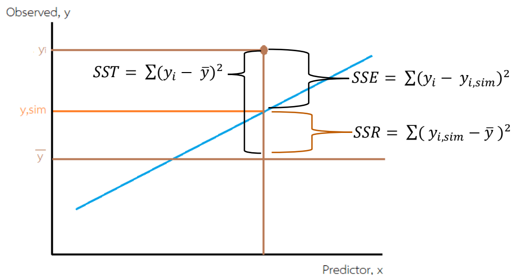
รูปที่ 5.3.2-1 การประมาณค่าสำหรับการคำนวณค่า r^2
