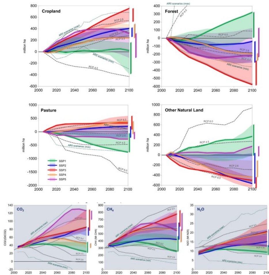
รูปที่ 4.4.1-2 การใช้ประโยชน์ที่ดินและการปล่อยก๊าซเรือนกระจกของแต่ละสถานการณ์ SSPs
