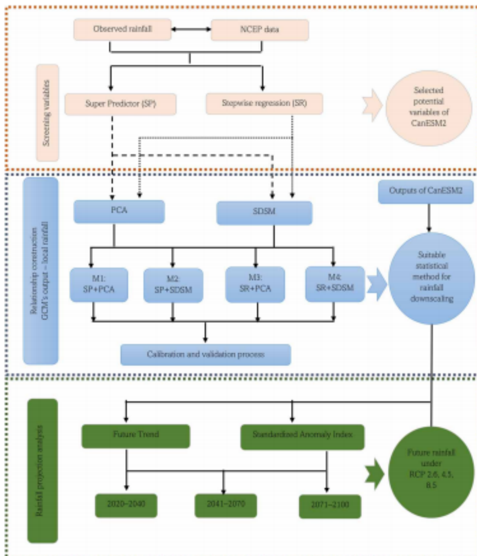
รูปที่ 5.4.3-1 ตัวอย่างการทำงานการประยุกต์ใช้วิธีการทางสถิติร่วมกันจากงานวิจัยของ Onarun et al (2023)
