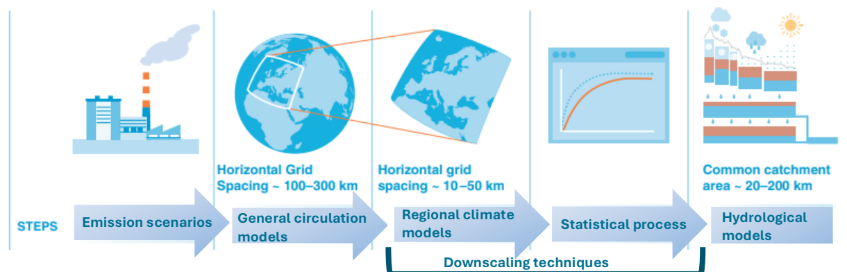
รูปที่ 6.3-1 ขั้นตอนการประเมินผลกระทบของการเปลี่ยนแปลงสภาพภูมิอากาศที่มีต่อปัจจัยทางด้านอุทกวิทยา
