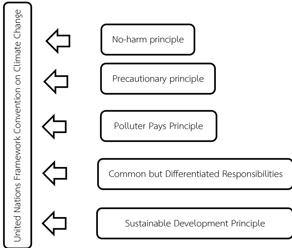
รูปที่ 1.5.1-1 หลักการของกรอบอนุสัญญา UNFCCC
