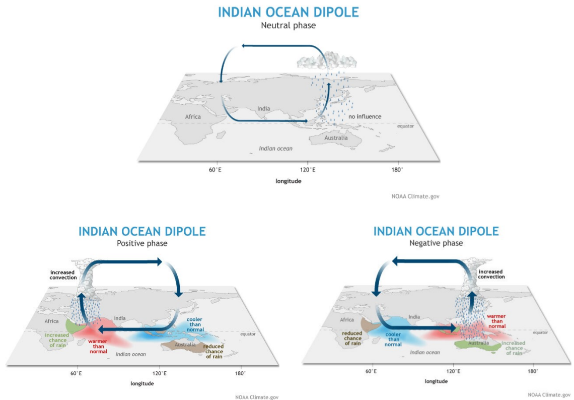
รูปที่ 2.4-1 สถานะของ Indian Ocean Dipole
