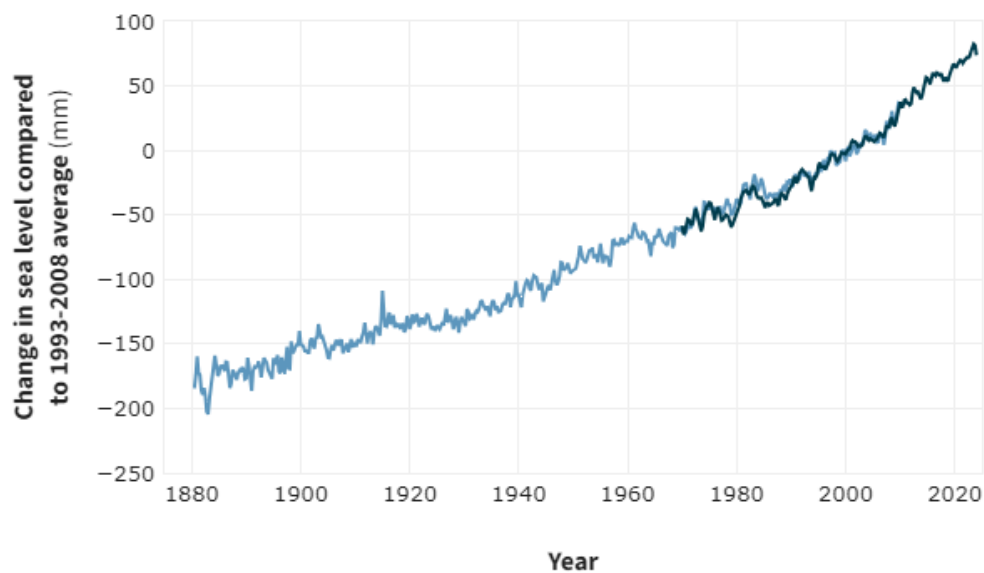
รูปที่ 1.3.2-2 การเปลี่ยนแปลงของระดับน้ำทะเลรายปีเมื่อเปรียบเทียบกับค่าเฉลี่ยในช่วงปี 1993-2008
