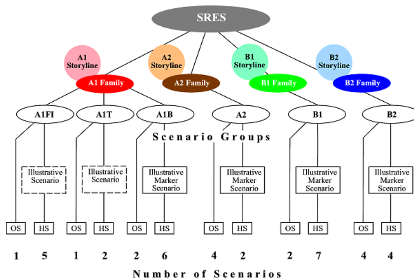
รูปที่ 4.2.1-1 SRES emission scenarios
