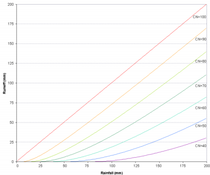
รูปที่ 3.1.1-1 ความสัมพันธ์ระหว่างปริมาณน้ำท่าและปริมาณฝนในแต่ละ CN
