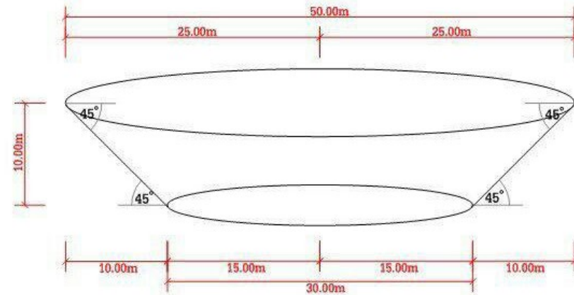
รูปด้าน บ่อกักเก็บและส่งน้ำ ขนาดเส้นผ่านศูนย์กลาง 50 เมตร
