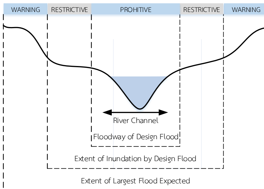
รูปที่ 4-2 รูปตัดขวางของพื้นที่ลุ่มน้ำซึ่งมีการจัดเขตพื้นที่ตามที่ระบุ
