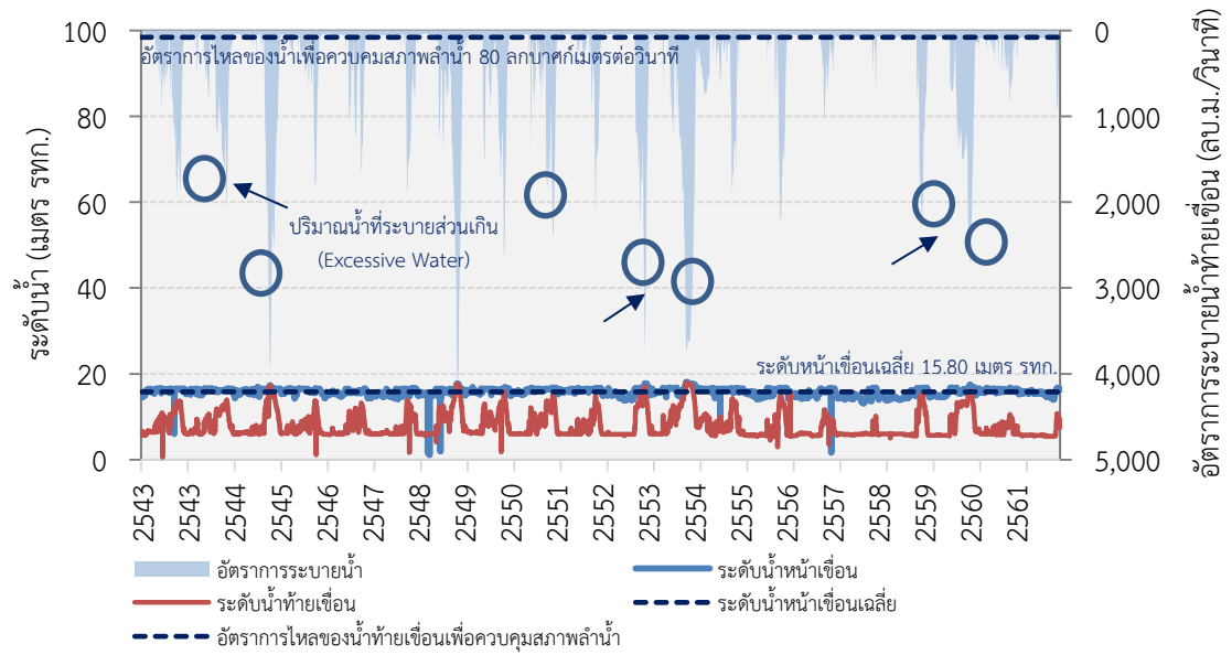
รูปที่ 3 แนวทางการจัดสรรน้ำของเขื่อนเจ้าพระยาตั้งแต่ปี พ.ศ. 2543-2562
