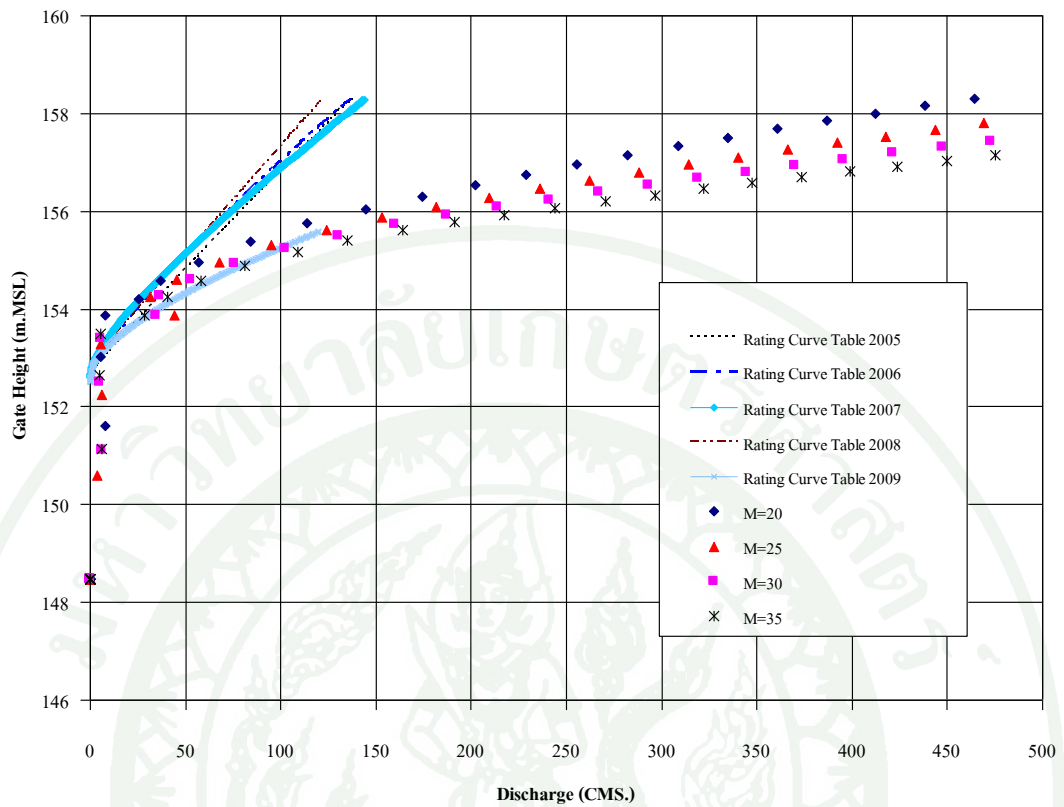
ภาพที่ 28 ผลการเปรียบเทียบแบบจำลอง MIKE11- HD ในแม่น้ำอุน โดยใช้ Rating Curves ที่สถานี 022901
