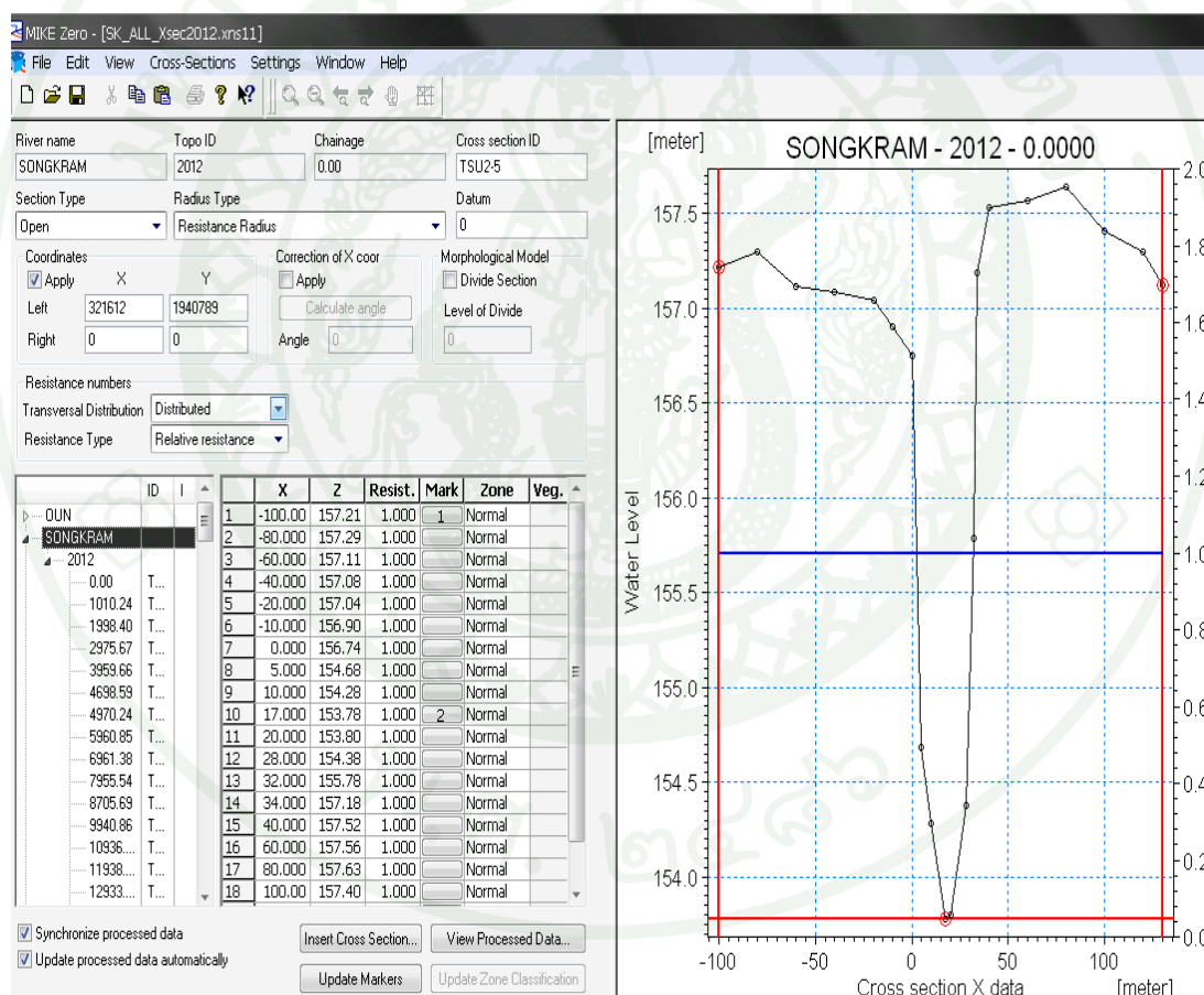
ภาพที่ 13 หน้าตัดรูปตัดลำน้ำของแม่น้ำสงครามในแบบจำลอง MIKE11- HD
