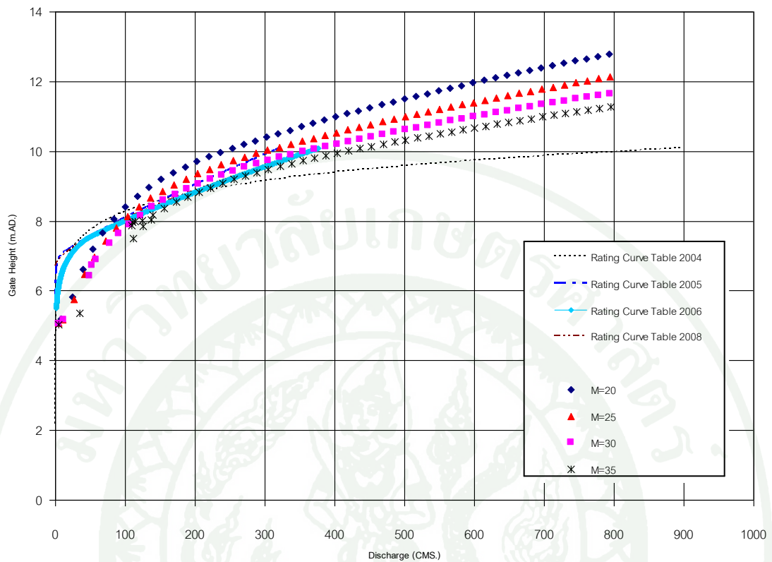
ภาพที่ 30 ผลการเปรียบเทียบแบบจำลอง MIKE11- HD ในหัวข้อนี้ โดยใช้ Rating Curves ที่สถานี 022701
