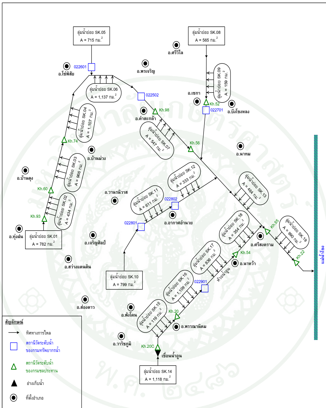
ภาพที่ 15 แผนภูมิแสดงระบบการไหลของน้ำในกลุ่มน้ำสงคราม (พื้นที่กลุ่มน้ำรวม 13,146 ตร.กม.)
