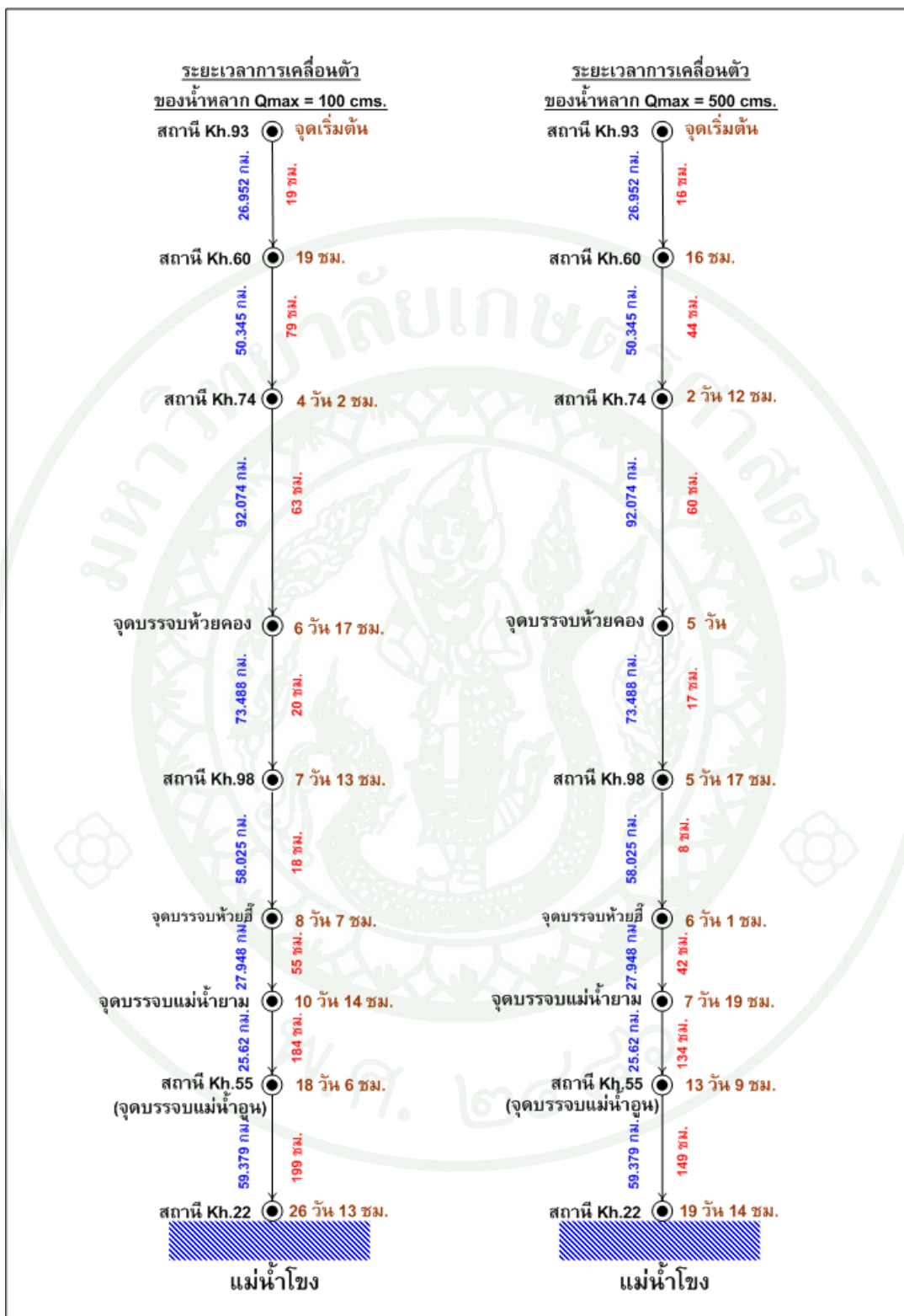
ภาพที่ 31 ระยะเวลาการเคลื่อนตัวของน้ำหลากที่ค่าอัตราการไหลสูงสุด 100 cms และ 500 cms
